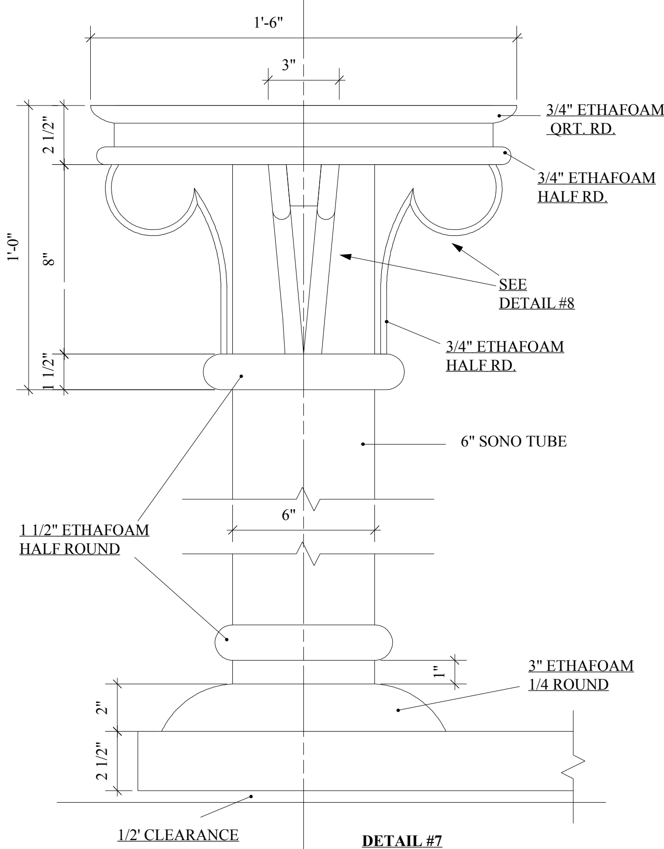
DETAIL #7 SCALE: 3"=1'-0"
