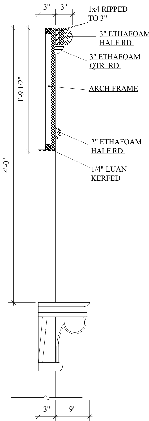
SECTION Z-Z' SCALE: 1 1/2"=1'-0"
