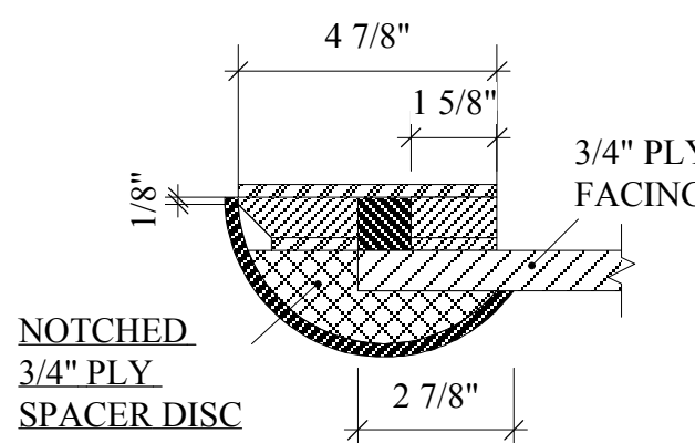
SECTION T-T' SCALE: 3"=1'-0"
