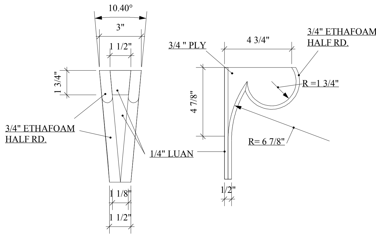
DETAIL #8 CAPITOL DETAIL SCALE: 3"=1'-0"
