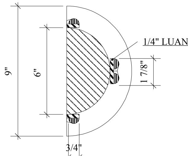
SECTION Y-Y' SCALE: 3"=1'-0"
